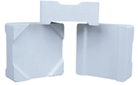
FIRIN KEPİ 100,5x100,5 mm Ürün Kodu: SRK015
